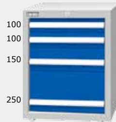
EA-7042 重量型工具柜 工具柜尺寸： H700 x W566 x D607 抽屉荷重100kg 详见P48~51 抽屉配件： 第一层配置标准分类盒， 其他层配置标准隔板
